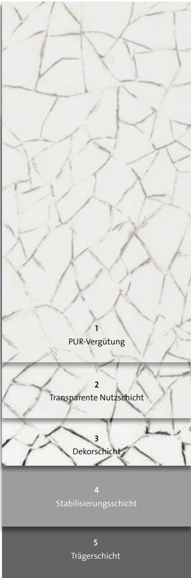
Aufbau EXPONA COMMERCIAL
